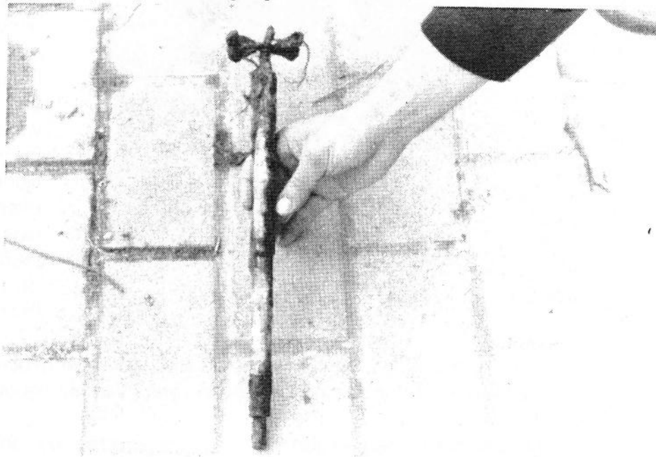
Neusbuis van Franse oorsprong voor vliegtuigbom TYPE H
